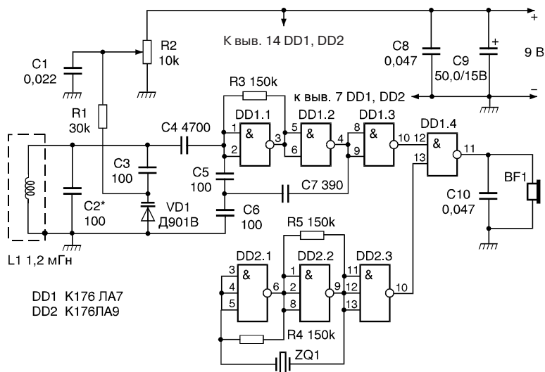
Рис. 5.15. Принципиальная схема металлоискателя повышенной чувствительности
