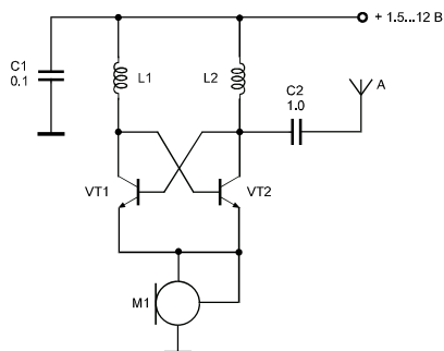
Рис. 2.30. Принципиальная схема микропередатчика со стабилизацией тока
