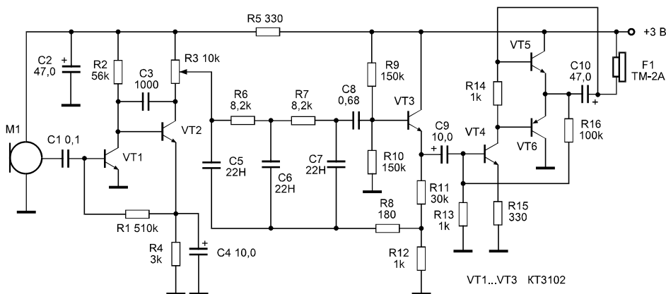
Рис. 2.4. Схема чувствительного микрофона с усилителем
