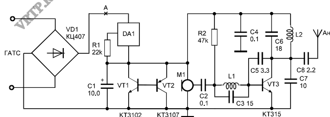
Рис. 3.30. Принципиальная схема радиомикрофона-радиотранслятора с питанием от телефонной линии
