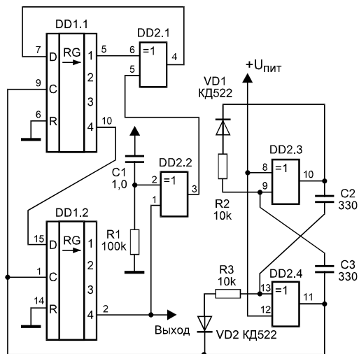
Рис. 2.22. Принципиальная схема цифрового генератора шума
