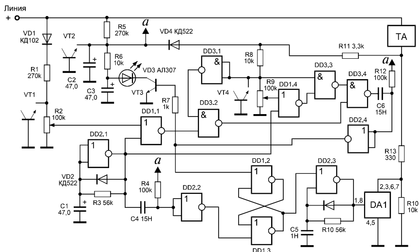
Рис. 3.12. Принципиальная схема активного индикатора состояния линии
