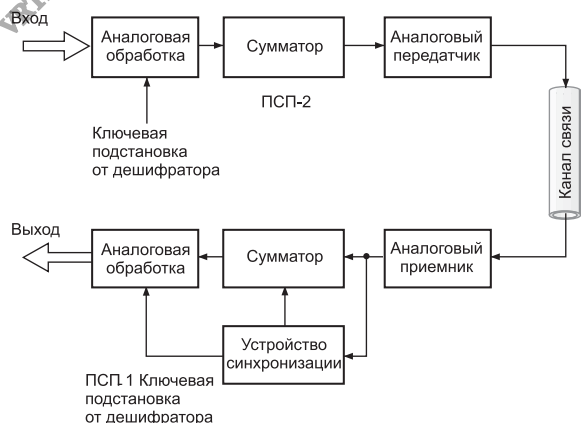
Рис. 3.36. Структурная схема маскиратора речевого сигнала заградительной помехой
