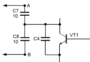
Рис. 3.28. Использование линии связи в качестве антенны
