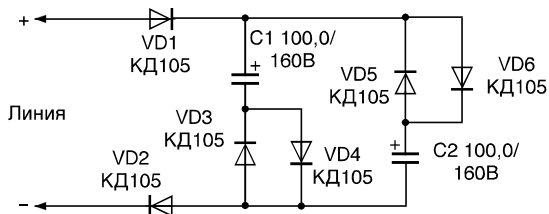
Рис. 3.13. Схема простейшего защитного устройства
