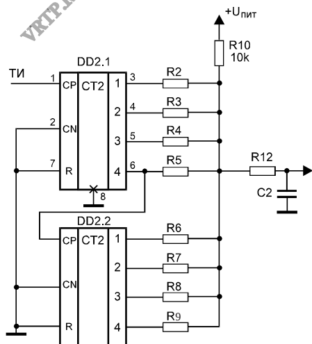
Рис. 2.79. Использование микросхемы K561ИЕ10
