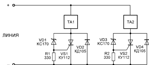
Рис. 3.16. Принципиальная схема блокиратора на аналоге динистора
